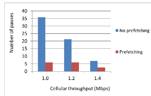
Fig. 6. Video QoE
